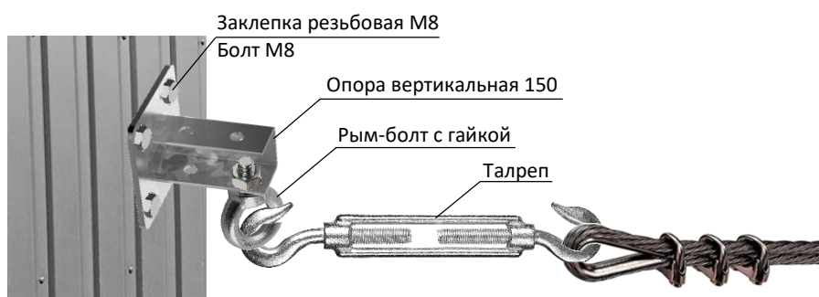
Рис. 7.1.4 Пример узла крепления троса к профильному листу
