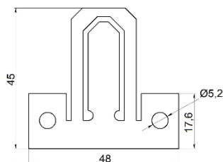
Рис. 3.3.3 Держатель ДМОУ-1К-М
