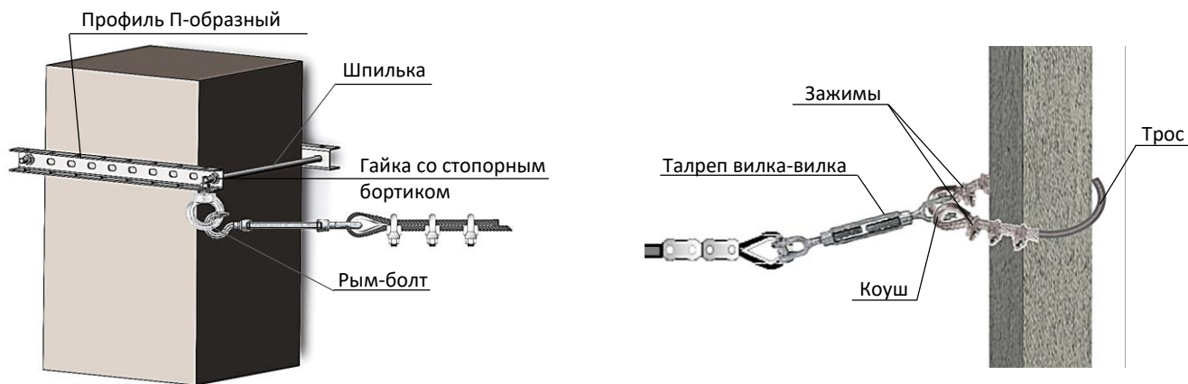
Рис. 7.1.3 Примеры узлов крепления троса к опорам
