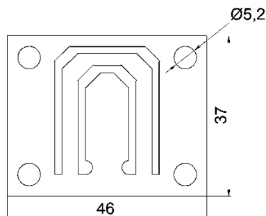
Рис. 3.3.1 Держатель ДМОУ-1К
