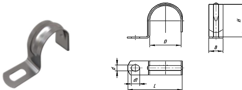
Рис. 3.4.1 Скоба металлическая однолапковая
