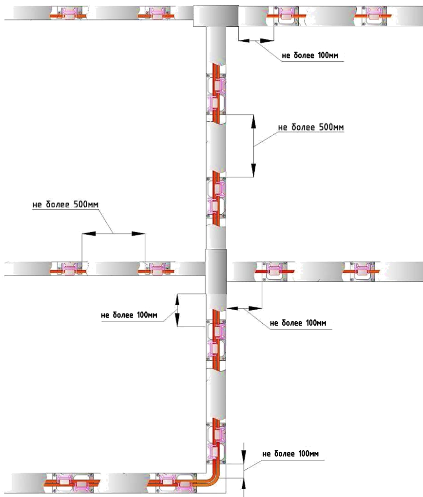
Рис. 2.3.1 Схема монтажа ОКЛ «ПожТехКабель РТК-Line-КК»
