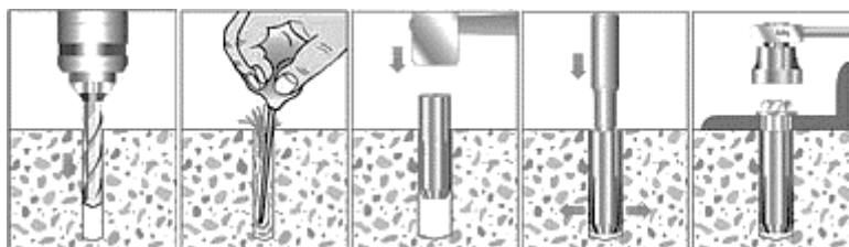
Рис. 3.8.2 Последовательность монтажа
